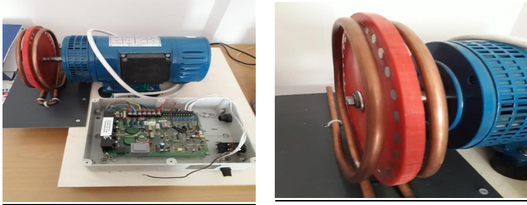
Şekil 1. Proje prototipinin görünüşleri
